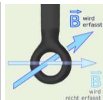
Bild 11: Die Magnetfeldsonde MS 02 erfasst Magnetfeld orthogonal zur Sondenöffnung /zum Sondenschaft.
