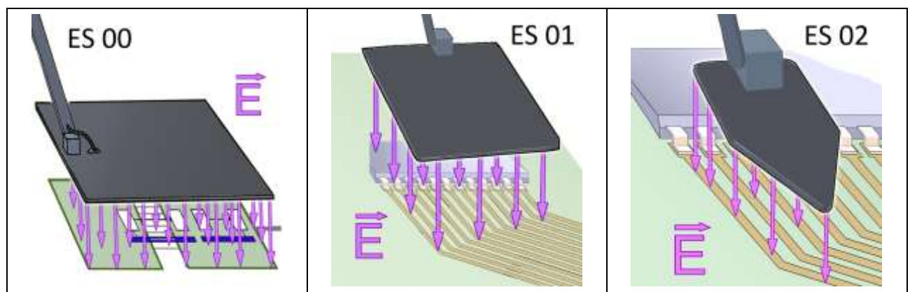
Bild 39: Feldquellen ES 00 - 02 mit großem Feld zur Beaufschlagung von Leiterzugschleifen um 10 cm.
