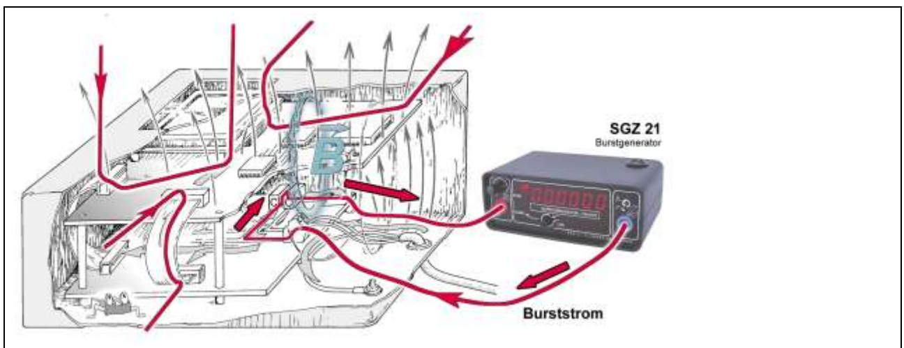
Bild 19: Zweipoliges Einspeisen mit dem SGZ 21 in den Prüfling
