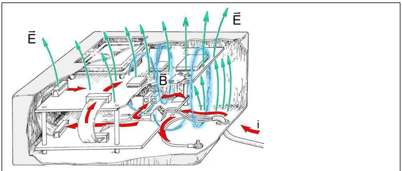
Bild 17: Störstromwege im Prüfling bei einer Burstprüfung
