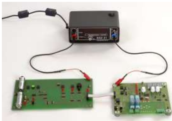
Bild 26: Einspeisen von Störstrom zweipolig über den Steckverbinder zweier Baugruppen. Die Kontaktierung erfolgt jeweils an Masse der Baugruppen.
