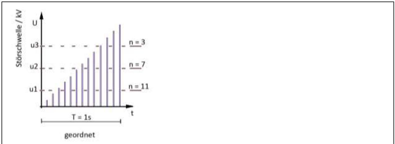
Bild 12: Rampenförmiger Anstieg der Störimpulse des SGZ 21. Störschwellenüberschreitungen n bei unterschiedlich hohen Störschwellen u .
