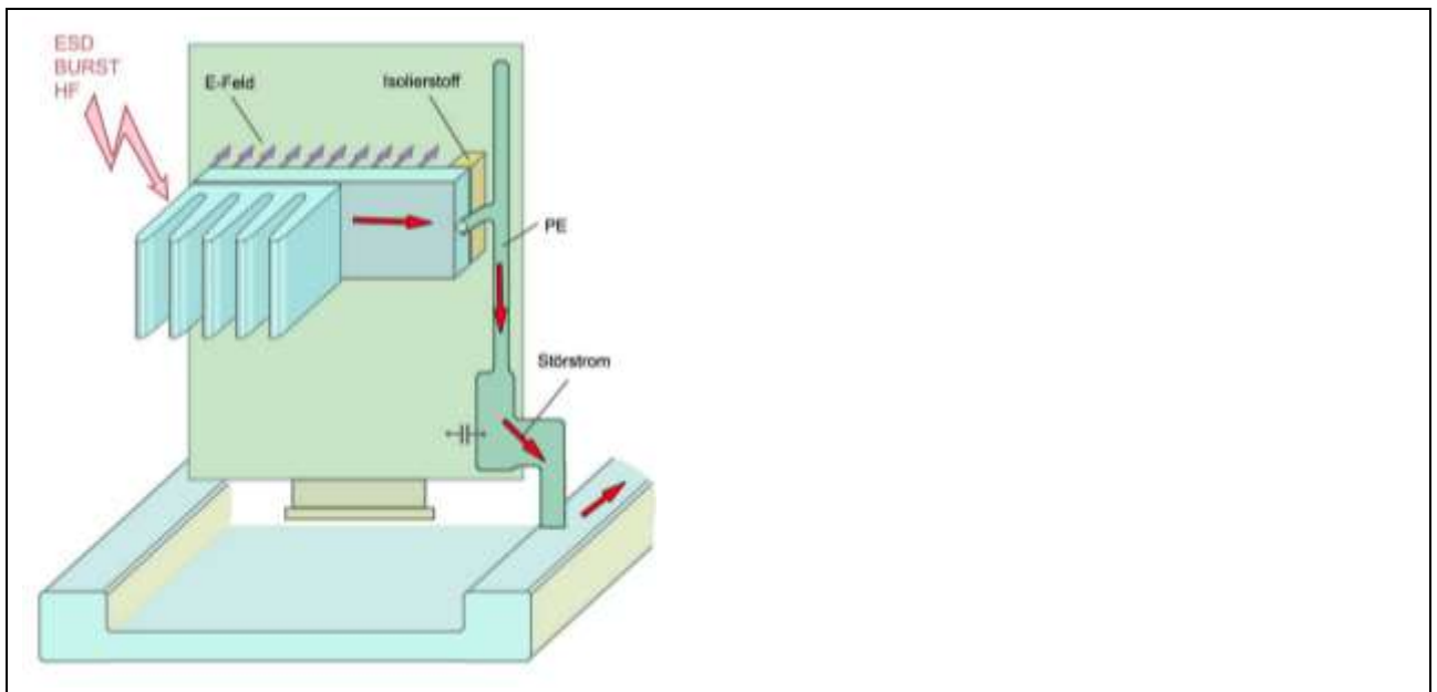
Bild 30: Praktisches Beispiel für eine Baugruppe, die vom elektrischen Feld eines benachbarten Konstruktionsteils beeinflusst wird.
