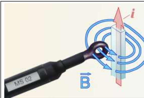
Bild 10: Messung von Magnetfeld mit der Sonde MS 02
