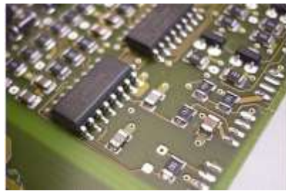
Bild 28: Masse-Lage anfräsen, Kontaktstift anlöten, Generatorkabel an den Kontaktstift mit den Mikro-Klebs ankleben und damit Störstrom leitungsgebunden in Masse einspeisen
