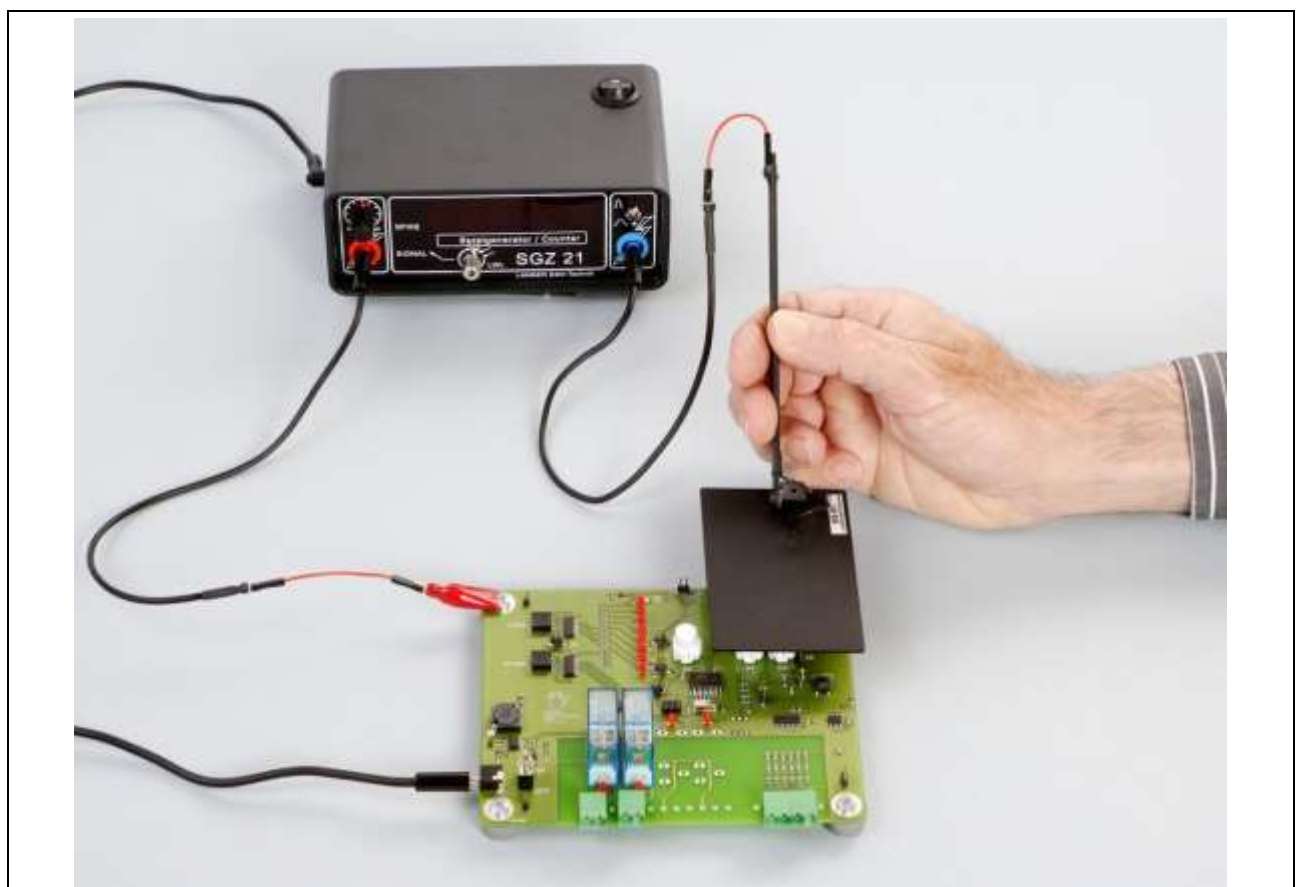
Bild 41: Die E-Feldquelle wird zur Beaufschlagung von Leitungen schrittweise der Baugruppe genähert.
