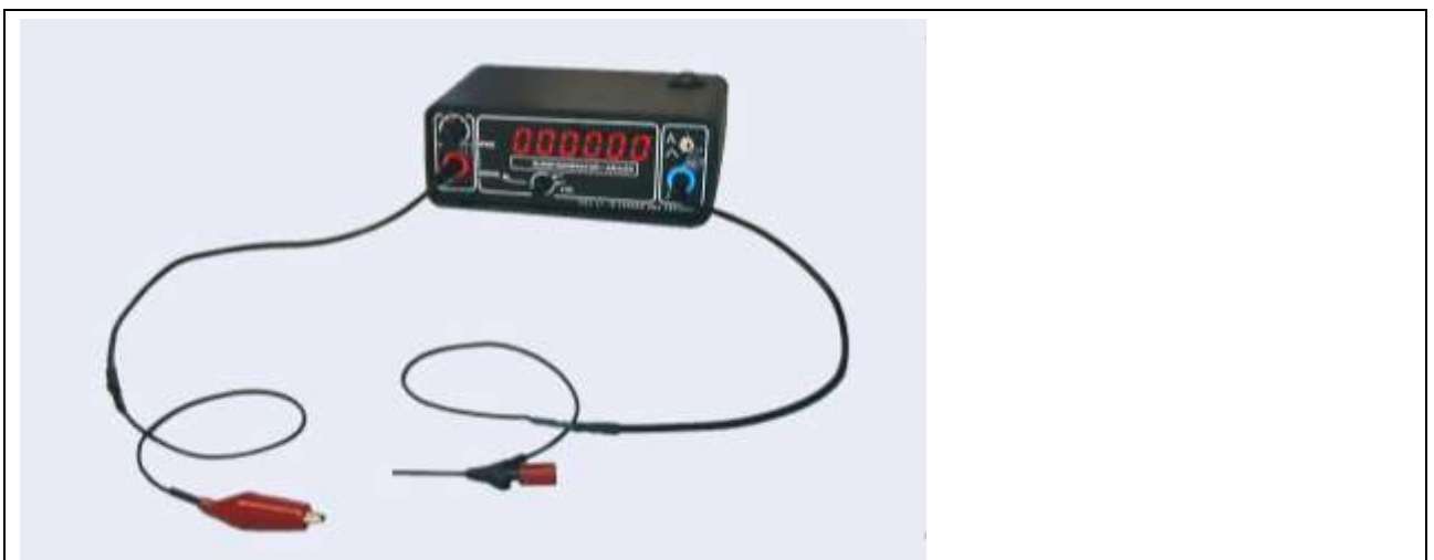
Bild 5: SGZ 21 mit angeschlossenen Generatorkabeln, einer Krokoklemme und einem Mikro-Kleps
