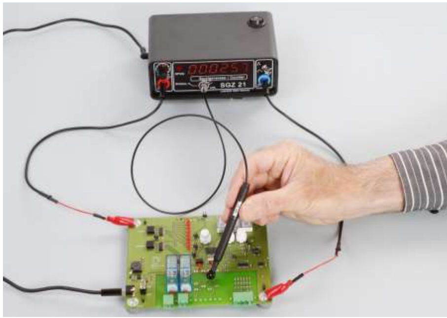
Bild 45: Messaufbau zur Magnetfeldmessung mit der Magnetfeldsonde MS 02
