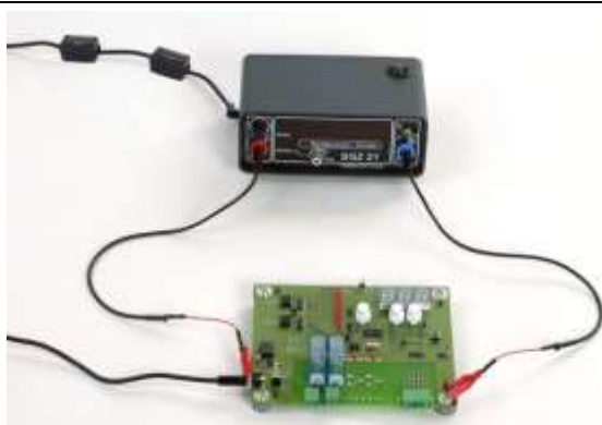
Bild 24: Einspeisen von Störstrom zweipolig über eine galvanische Trennstelle durch den Prüfling
