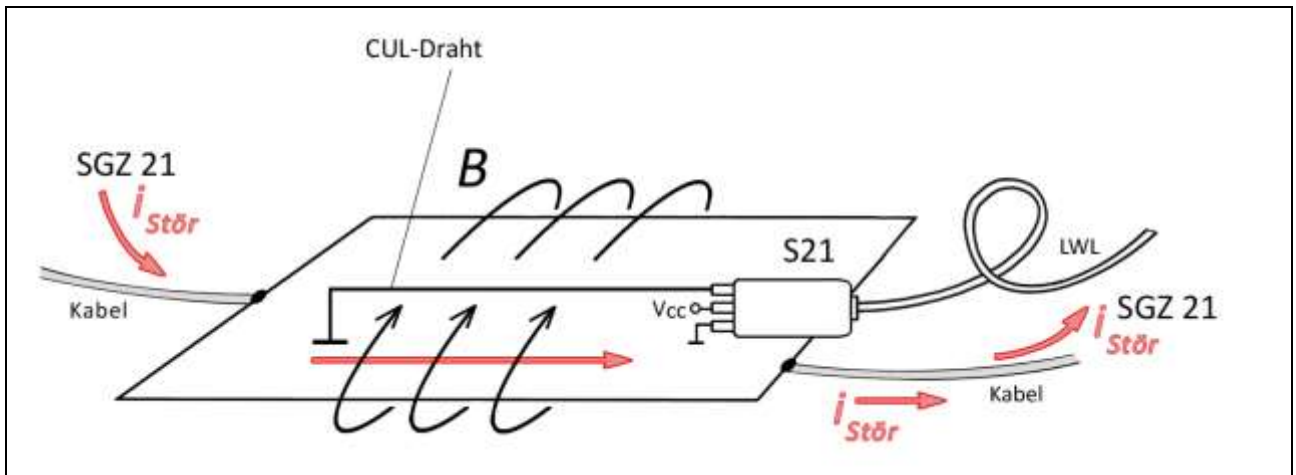
Bild 13: künstliche Magnetfeld-Störschwelle durch Einbringen des Sensors S21 mit Kupferlackdraht als Leiterzugnachbildung
