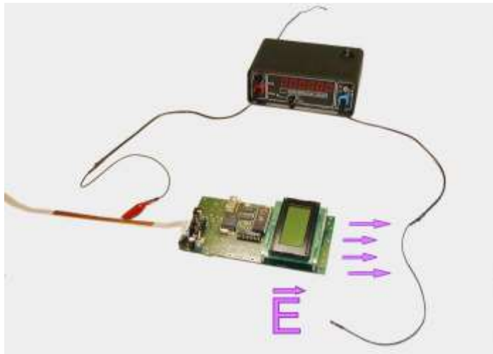
Bild 29: Einpolige Einspeisung des Störstroms mit dem Burst-Generator SGZ 21 erzeugt ein elektrisches Feld zum Gegenpol des Generators.
