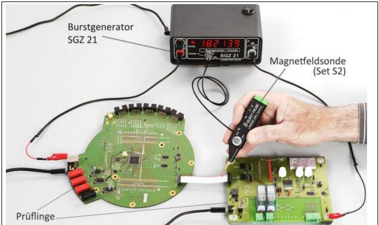
Bild 47: Messung von Störstrom in den einzelnen Adern der Flachbandleitung mit den Sonden des Set S2
