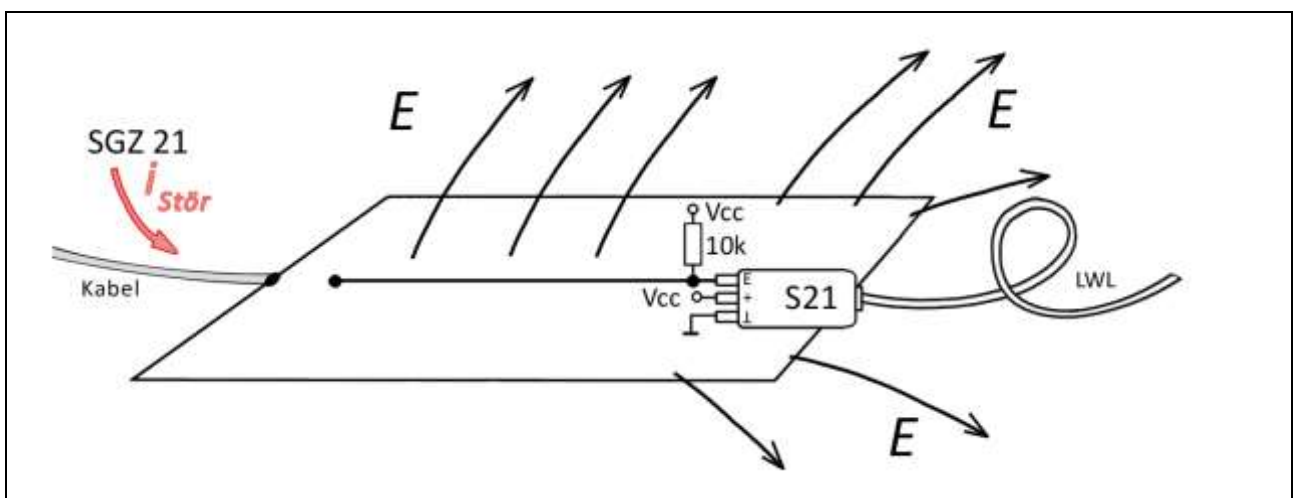
Bild 14: künstliche E-Feld-Störschwelle durch Einbringen des Sensors S21 mit Kupferlackdraht als Leiterzugnachbildung
